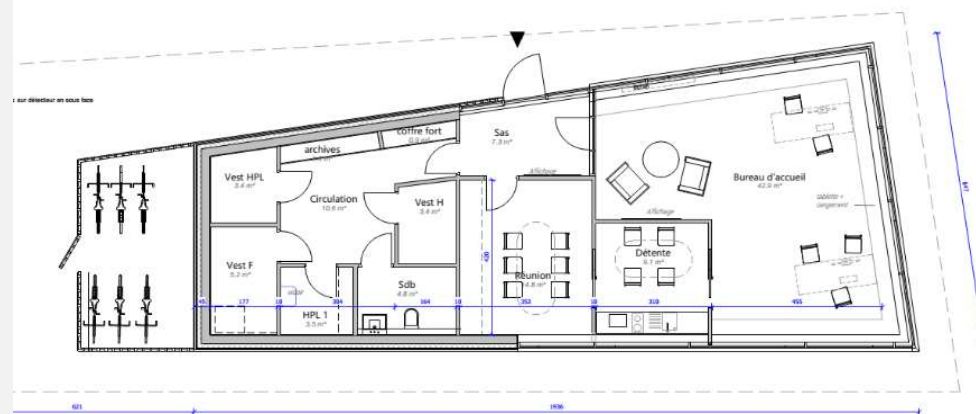
BATIMENT SUD : bureau du port ech : 1/100
